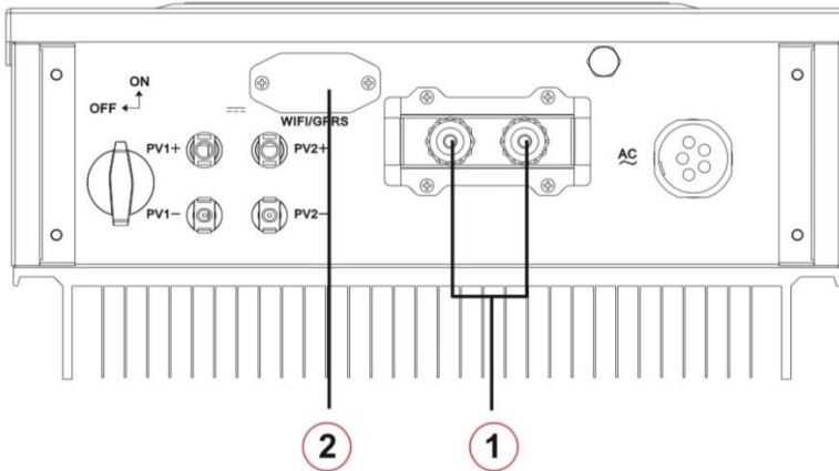
Kuva 4-5 WiFi/RS485 kuvaus
