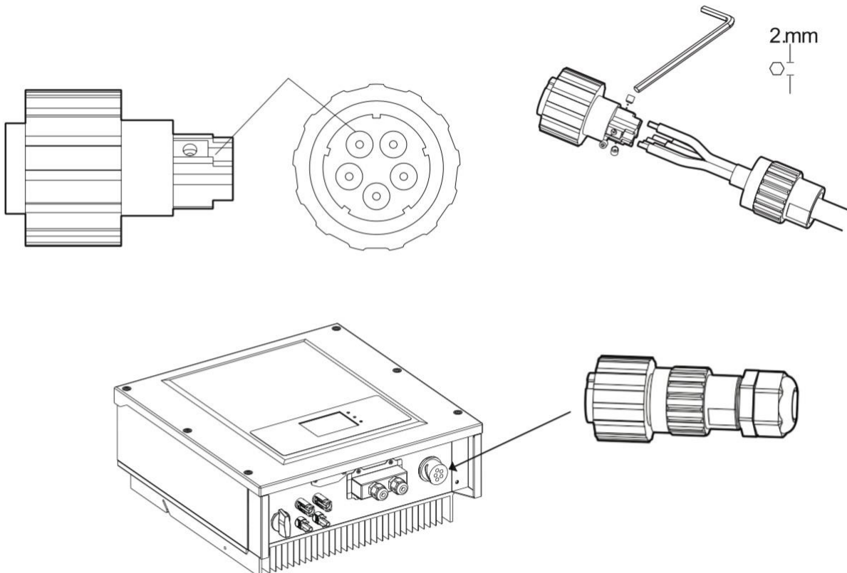
Kuva 4-4 Johtokytkennän kuvaus
