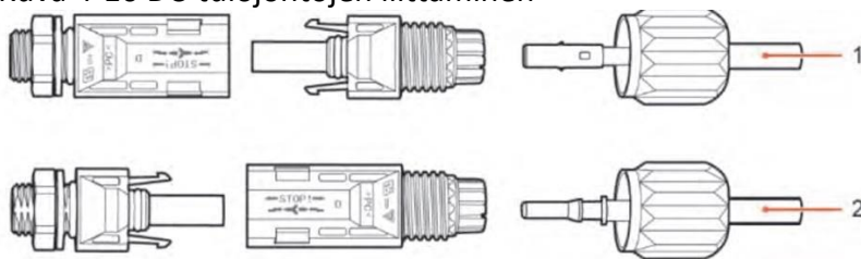
Kuva 4-16 DC-tulojohtojen liittäminen
