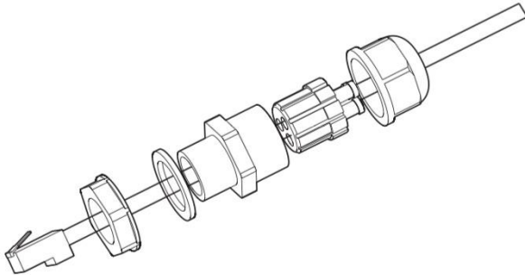
Kuva 4-8 RS485-kommunikaatiokaapeleiden kytkeminen (2)
