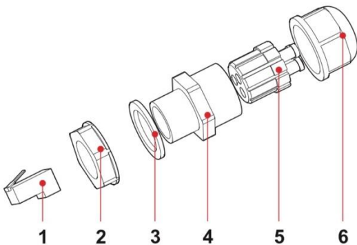
Kuva 4-6 Vesitiiviin RJ45-liittimen kuvaus
