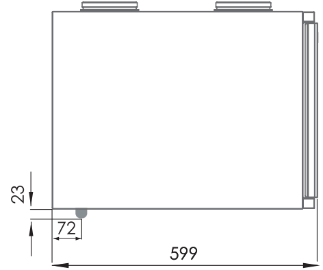
L/R-malli sivusta
